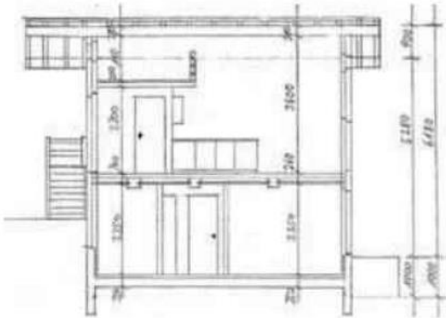
Schnitt
